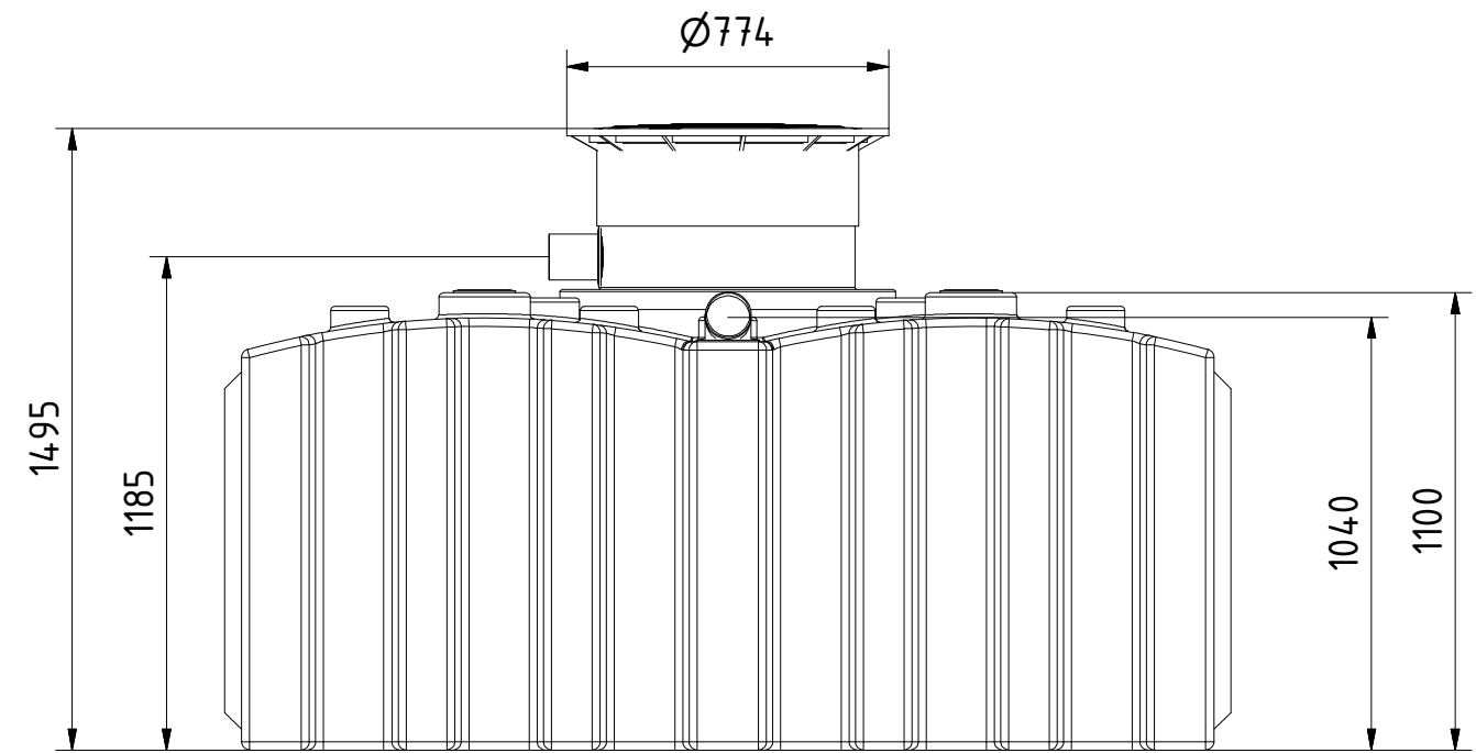
Frontansicht
